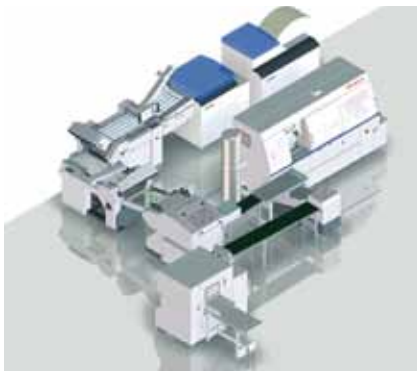
Sistema de encuadernación a partir de bobina. Con esta solución se pueden encuadernar libros con dato variable.
